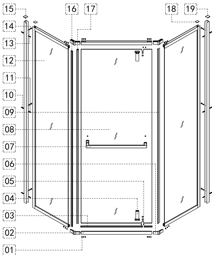
Gehäuse konfiguration / Enclosure configuration / Комплектация ограждения 90x90
